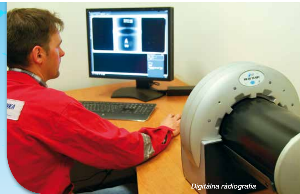
RTG prístroj
